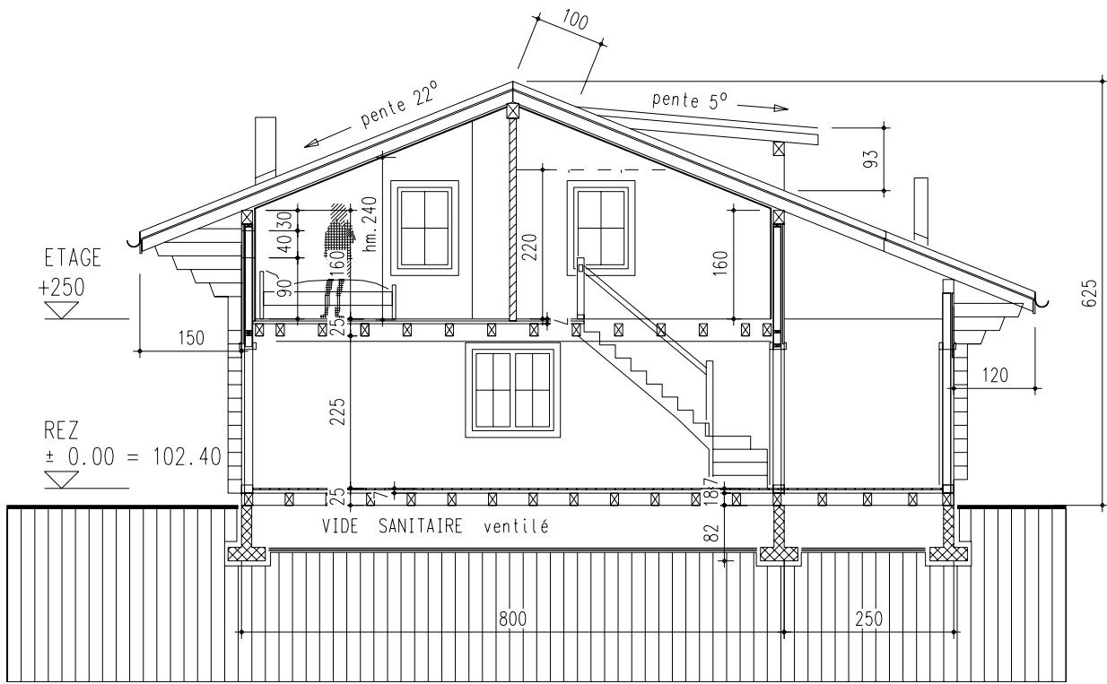
Coupe A-A
