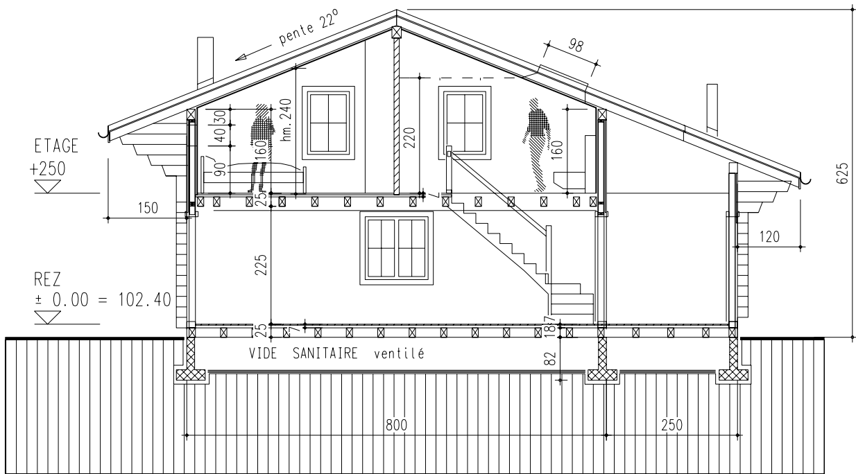
Coupe A-A
